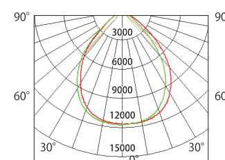
配光図
