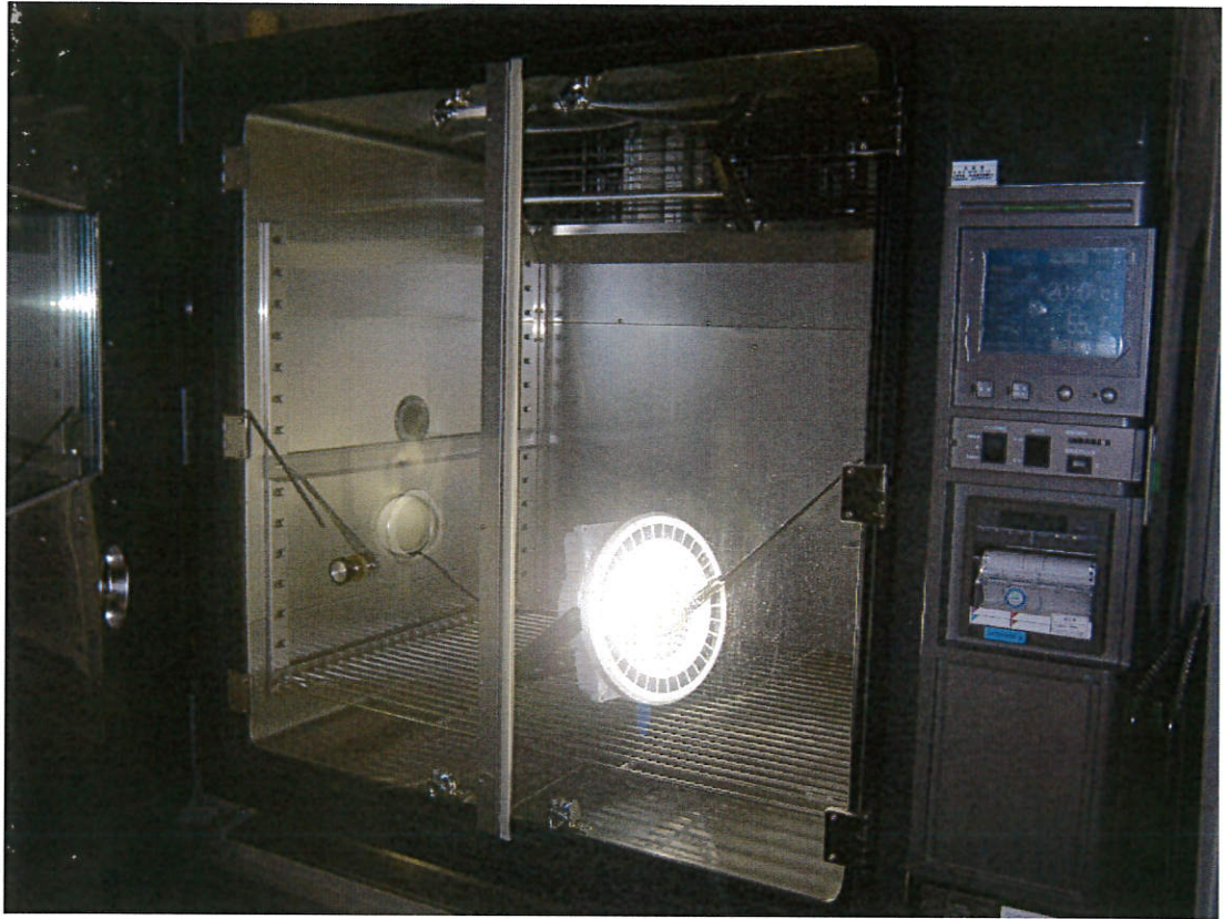
写真 2 温湿度サイクル試験の様子
